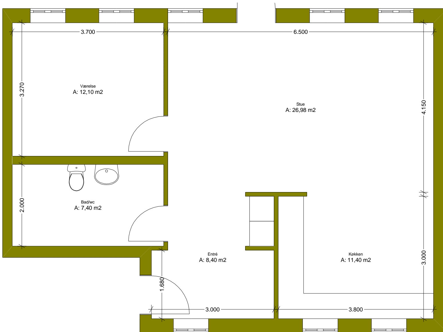
Stueplan
