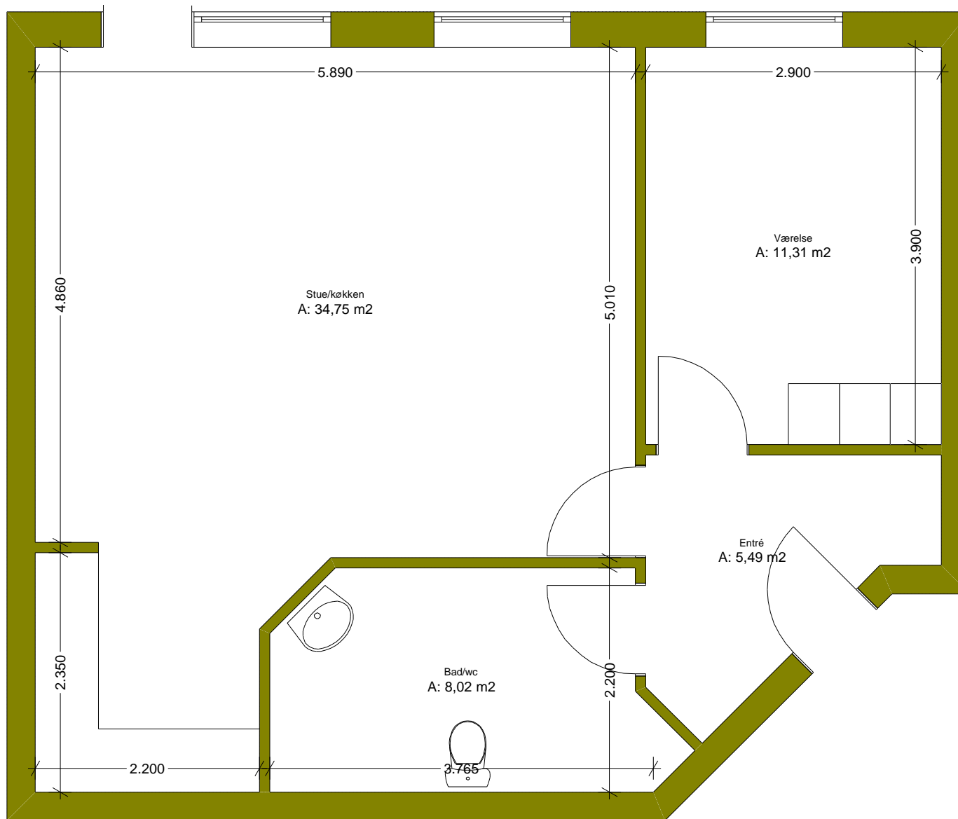
Stueplan
